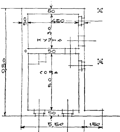
Plan d'une maison-type pour sinistrés.
